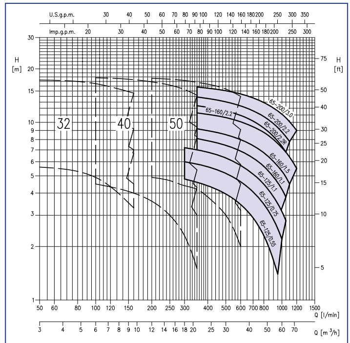
4 Poles - 50 Hz
